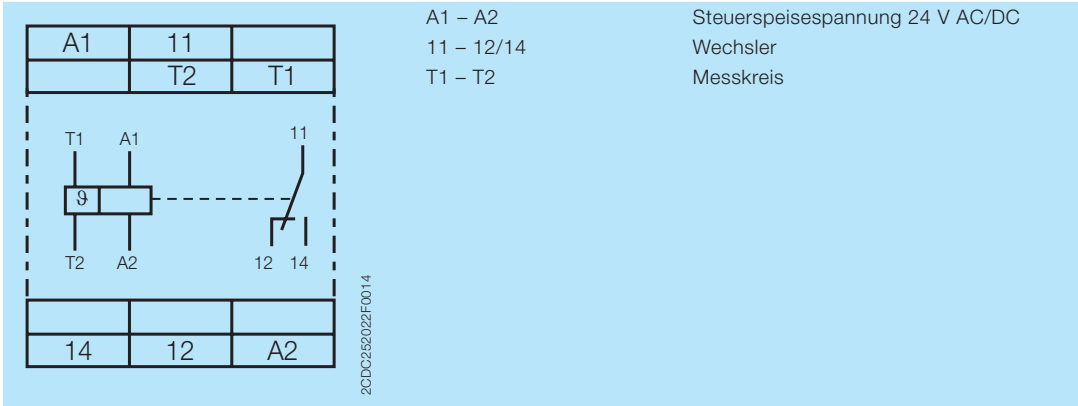
Anschlussbild CM-MSS.12
