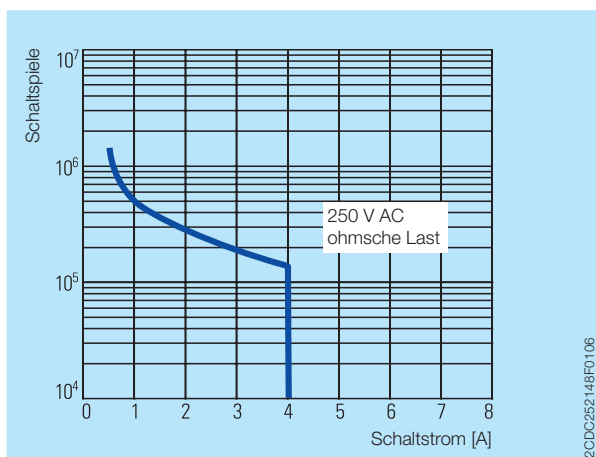
Kontaktlebensdauer / Anzahl der Operationen N 220 V 50 Hz 1 AC, 360 Operationen/h
