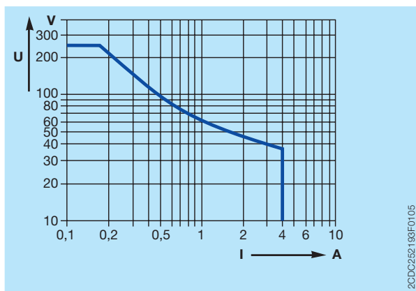
DC-Last (ohmsch)
