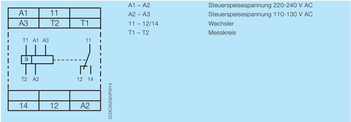
Anschlussbild CM-MSS.13
