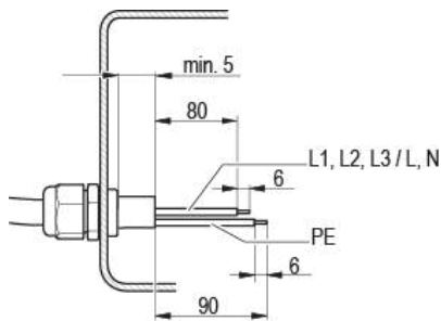
Abb. 1: Empfohlene Abmantellungsgrößen in mm (innerhalb Klemmkasten)
