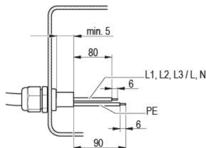
Abb. 1: Empfohlene Abmantellungslängen in mm (innerhalb Klemmkasten)
