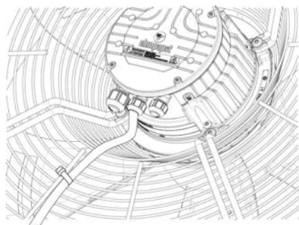
Abb. 2: Liegend eingebauter Ventilator, Verlegung des Kabels als Wassersack.
