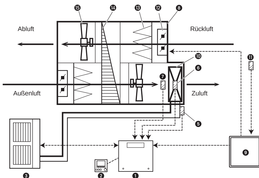
Beispiel (1-1): Steuerungsart MANUAL STEP *1
