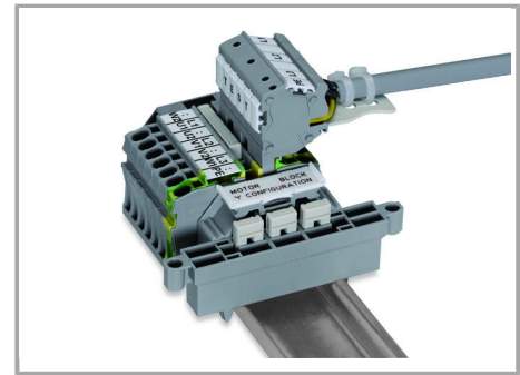
Motoranschluss-Klemmenblock
