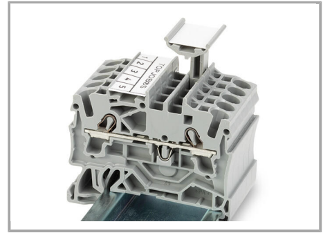
TOPJOB®S-Gruppenschildträger (2009-193) hier bestückt mit Beschriftungstreifen, verwendbar für alle TOPJOB®S- Reihen клемmen der Serien 2000 bis 2016.
