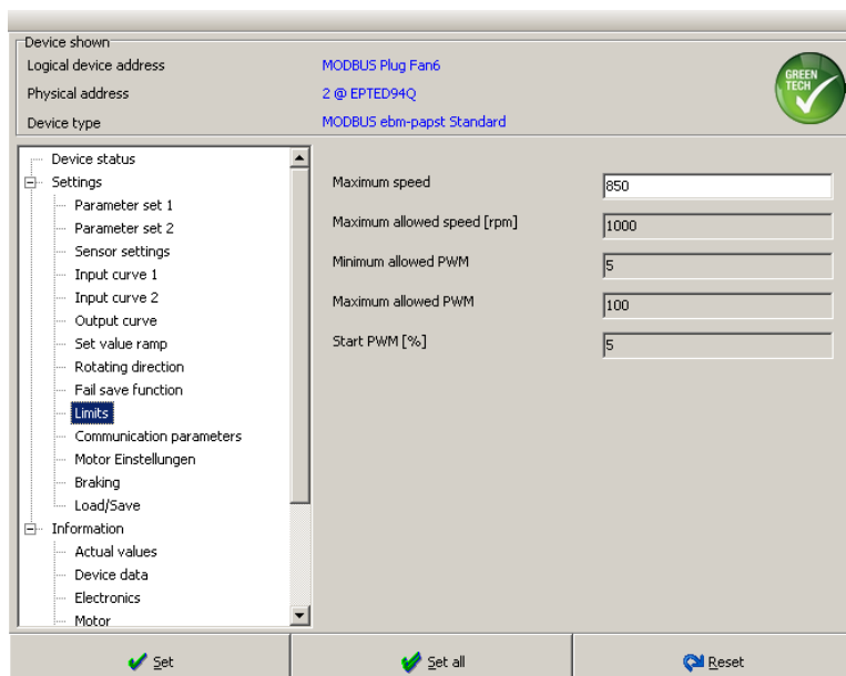
Fig. 13: Limit values
