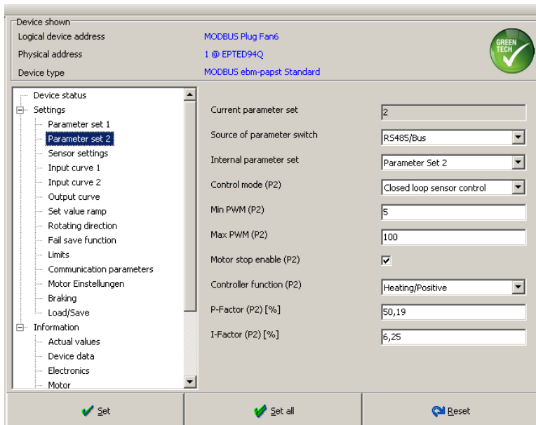
Fig. 59: Parameter set 2
